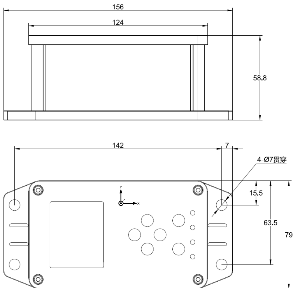
图示 6-1 机械尺寸 (单位: mm)
