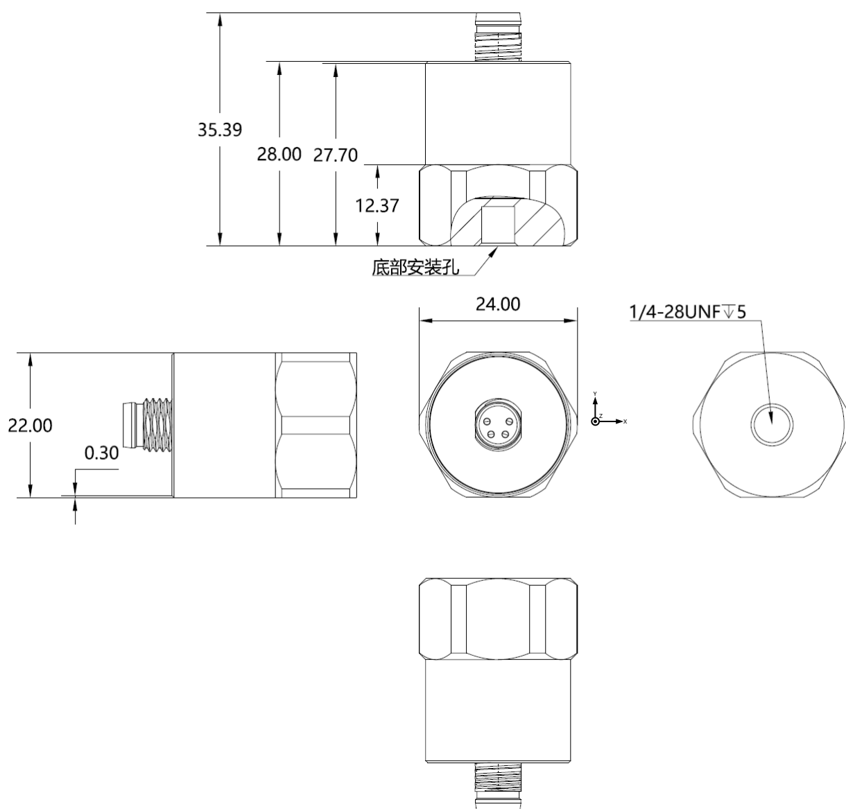
图示 6-1 机械尺寸 (单位: mm)
